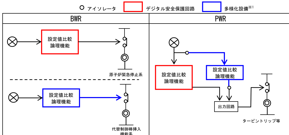
解説図 3.5.8-2 多様化設備と安全保護回路の分離例 (工学的安全施設作動機能)
