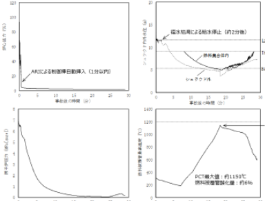
図 TRACGによるRHR出口配管破断 (給水継続) +デジタル安全保護系CCF解析例 (18分後HPCF手動起動を想定)
